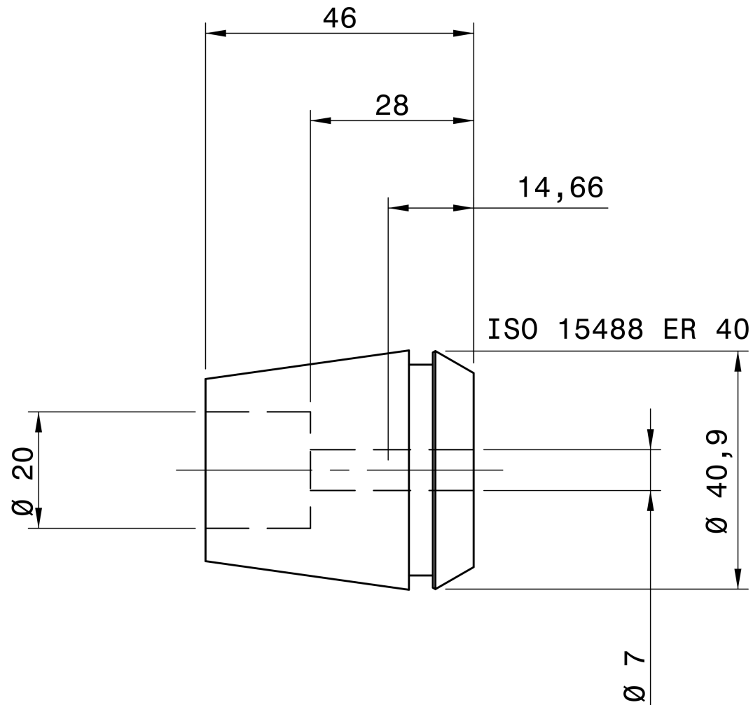
REGO-FIX 1140.07000
